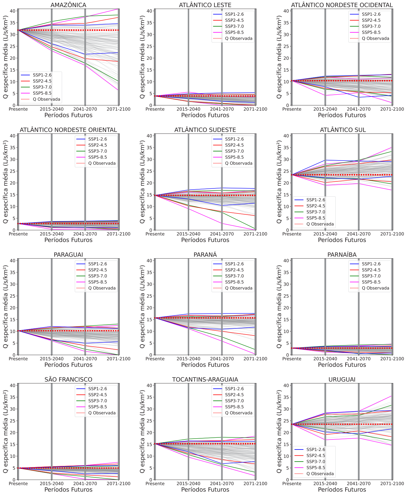
Figura 38 - Evolução das projeções futuras de QmIt específica incremental média de todos os MCGs e cenários de emissão para as 12 regiões hidrográficas brasileiras. As curvas coloridas são os limites de cada cenário.
