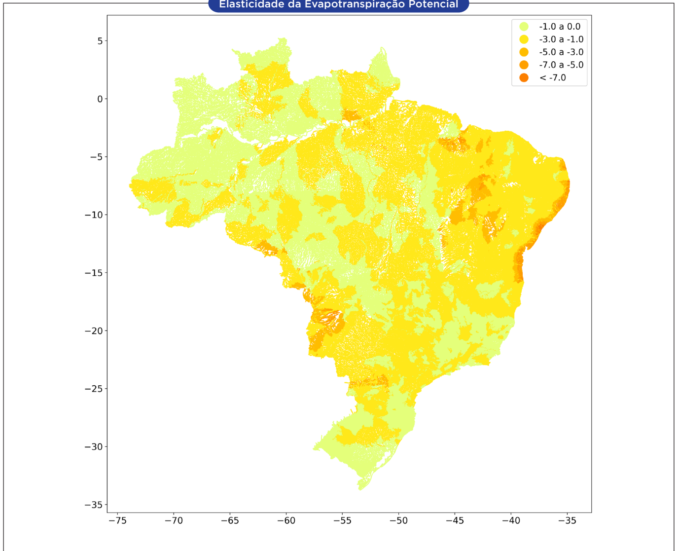
Figura 18 - Valores da elasticidade- evapotranspiração potencial ( \epsilon_2 ) com relação a vazão definidos para cada trecho ou ottobacia da BHO.
