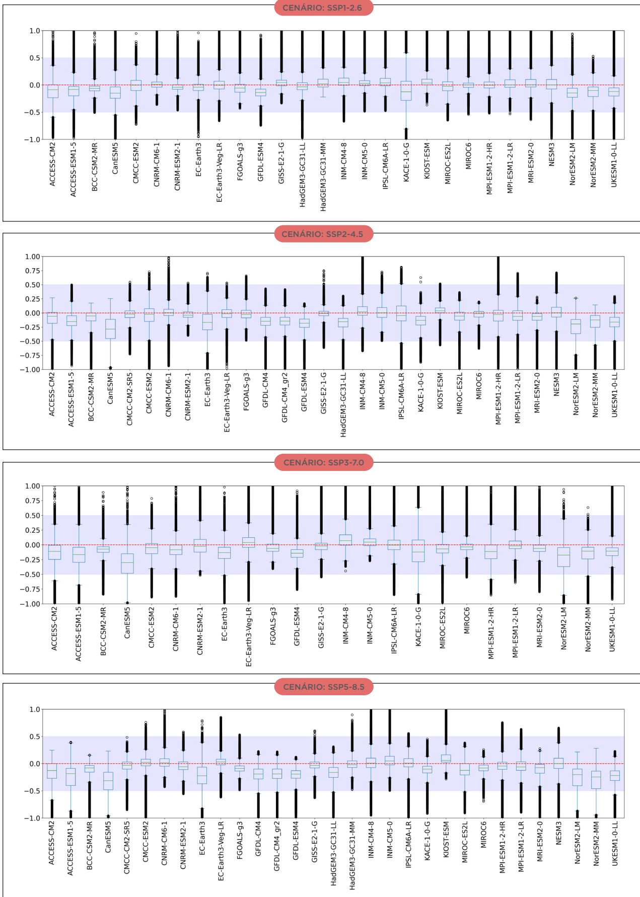
Figura 35 - Box Plot com todos os valores de Q_{mit} em todo o Brasil no período 2015-2040 considerando todos os MCGs e cenários de emissão.
