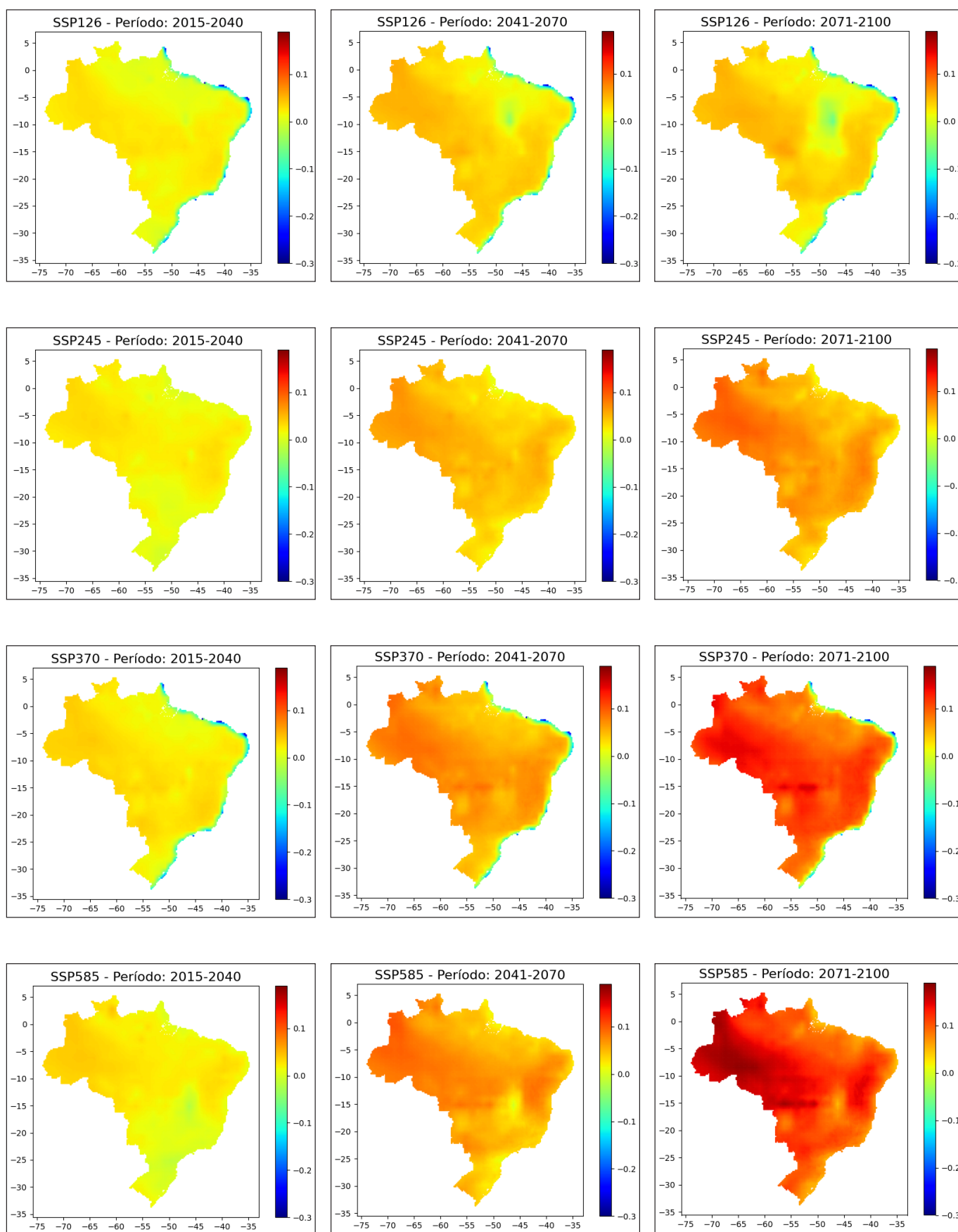
Figura 26 - Mapas da diferença relativa da EO para todos os períodos e cenários de emissão do MCG BCC-CSM2-MR.
