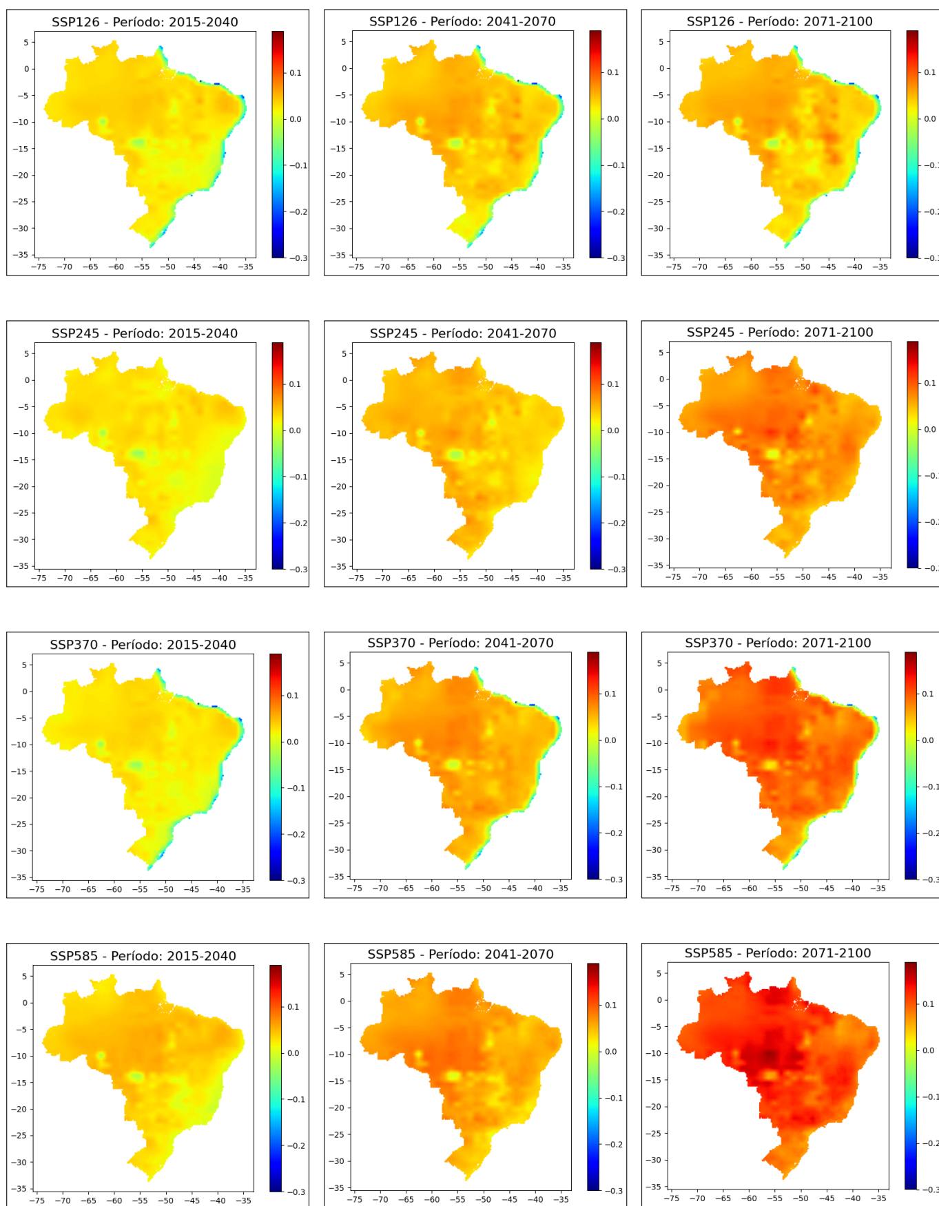
Figura 27 - Mapas da diferença relativa da E0 para todos os períodos e cenários de emissão do MCG NORESM2-MM.
