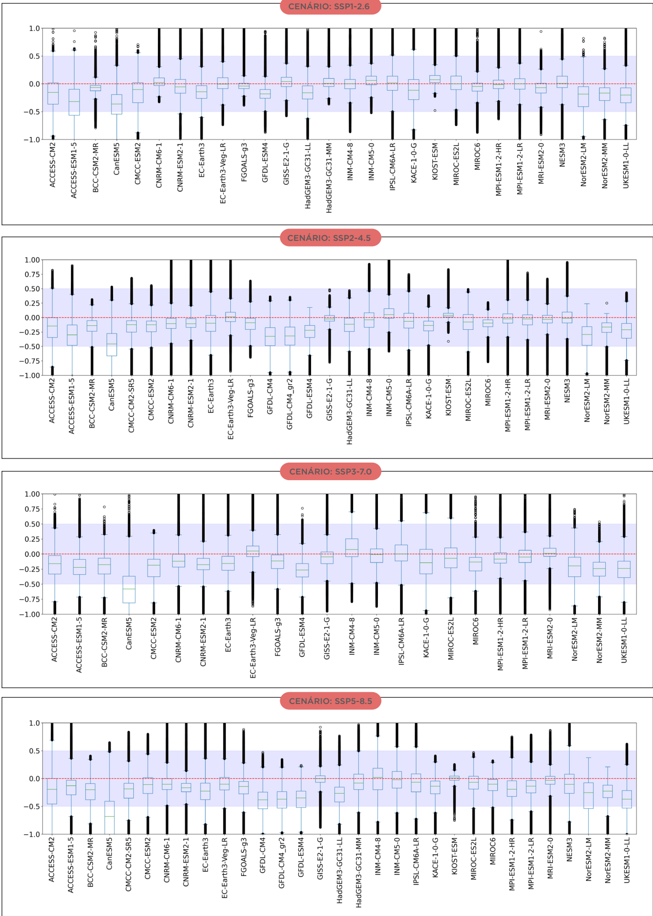
Figura 36 - Box Plot com todos os valores de Q_{m1t} em todo o Brasil no período 2041-2070 considerando todos os MCGs e cenários de emissão.
