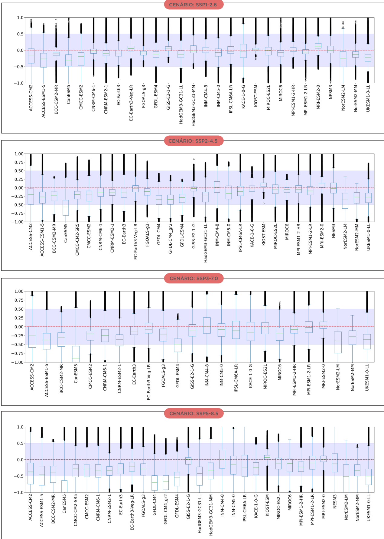
Figura 37 - Box Plot com todos os valores de Q_{mlt} em todo o Brasil no período 2071-2100 considerando todos os MCGs e cenários de emissão.
