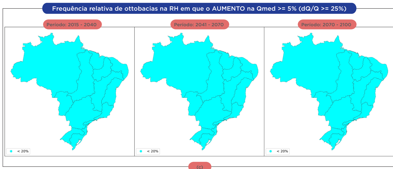
Figura 42 - Mapas do grau de convergência dos cenários climáticos para aumento na Qmlt em todos os períodos.
