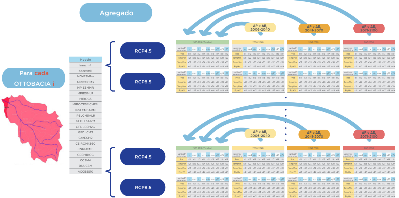
Figura 15 - Esquema de obtenção das mudanças percentuais na P e E para os diferentes horizontes temporais considerando os diferentes cenários de emissão e MCGs.
