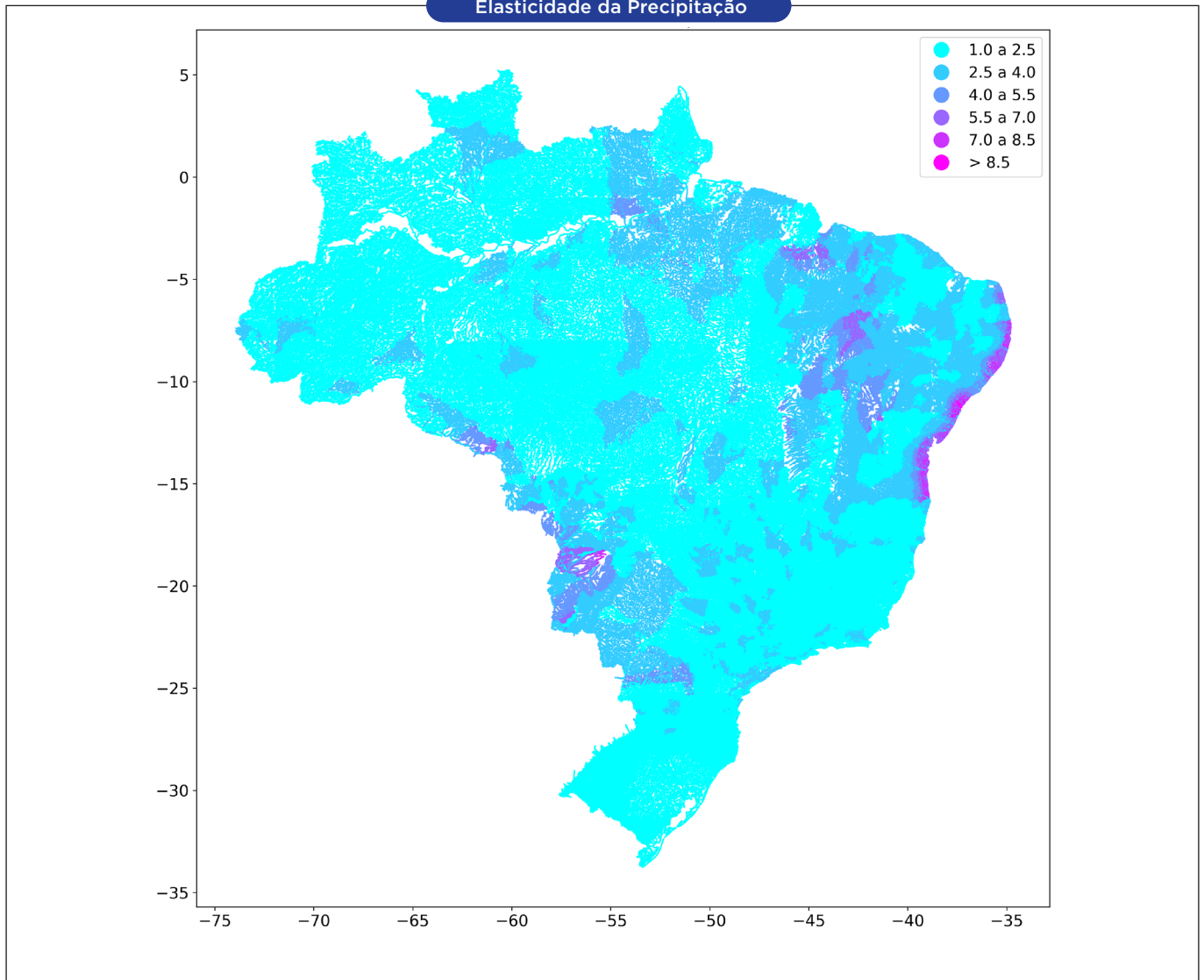
Figura 19 - Valores da elasticidade-precipitação ( \epsilon_1 ) com relação a vazão definidos para cada trecho ou subárea da BHO. tobacia da BHO.
