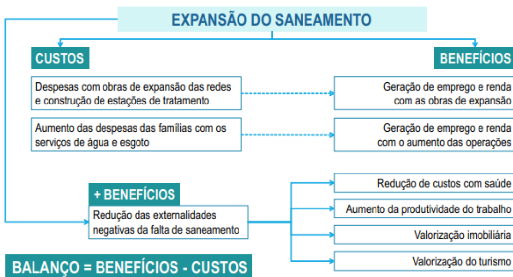
Figura 1 - Esquema metodológico
